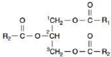
Gambar 3.3 Struktur Triasilgliserol (trigliserida) Sumber: Harper (2019)
