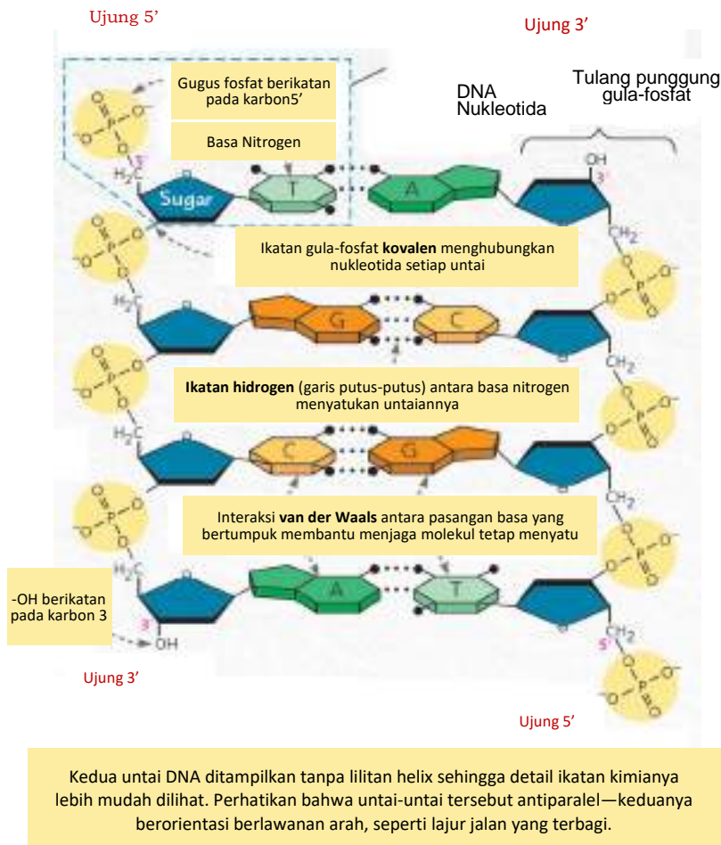
Gambar 5.3 Struktur DNA (Urry et al. , 2017)
