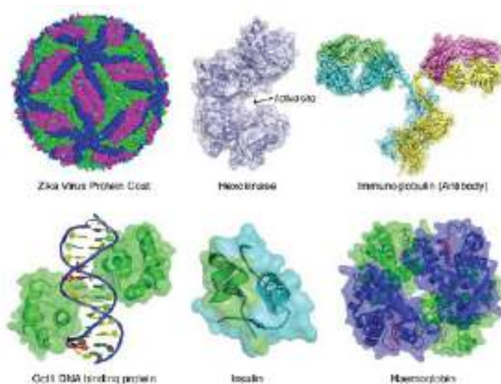
Gambar 4.4 Protein Mempunyai Beragam Struktur dan Fungsi Struktur protein sering dipandang sebagai model di mana untai- \beta direpresentasikan sebagai panah dan heliks- \alpha sebagai pita atau tabung. Misalnya, hemoglobin adalah
