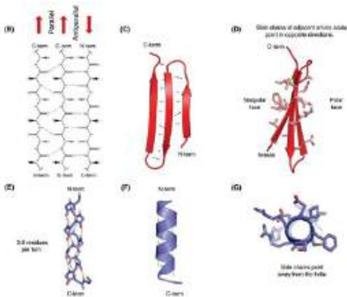
Gambar 4.3 (B) Gambar garis struktur kimia tulang punggung polipeptida dari tiga untai- \beta dalam lembaran- \beta . Ikatan hidrogen antara gugus -\text{CO} dan -\text{NH} rantai utama ditunjukkan sebagai garis putus-putus. Lembar paralel mengandung untai- \beta yang berjalan searah, sedangkan lembaran antiparalel mengandung untai- \beta yang berjalan berlawanan arah dengan tetangganya. (C) Representasi kartun (juga dikenal sebagai diagram pita) dari daerah lembaran- \beta antiparalel dari protein yang lebih besar. Dalam contoh ini, tiga untai- \beta dihubungkan oleh sebuah simpul pendek. Panah yang mewakili untai- \beta menunjuk ke arah ujung-C sesuai konvensi. Ikatan hidrogen yang menyatukan lembaran-lembaran tersebut ditunjukkan sebagai garis putus-putus. (D) Tampak samping dari lembaran \beta yang sama yang menunjukkan rantai samping residu individual. Atom-atom diwarnai dengan karbon merah muda, sulfur kuning, oksigen merah, dan nitrogen biru. Perhatikan bahwa residu di sisi non-polar sebagian besar tersusun dari residu yang mengandung karbon
