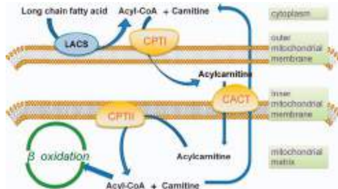
Gambar 8.3. Proses Transpor Asil-Koa ke Matriks Mitokondria (Qu et al., 2016)
