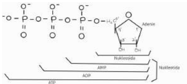
Gambar 5.2 Nukleosida monofosfat (AMP), difosfat (ADP), dan trifosfat (ATP).
