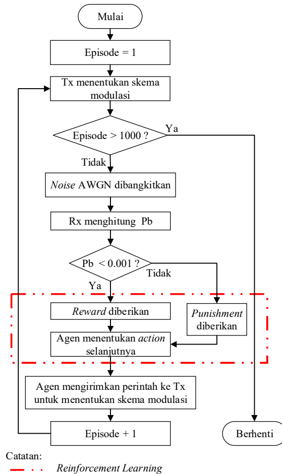
Gambar 4. Alur Simulasi
