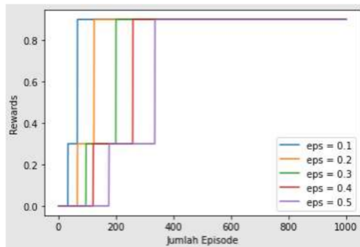
Gambar 7. Hasil Simulasi Kondisi Medium Noise
