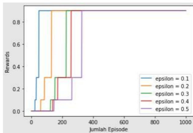
Gambar 5. Hasil Simulasi Seluruh Level Noise
