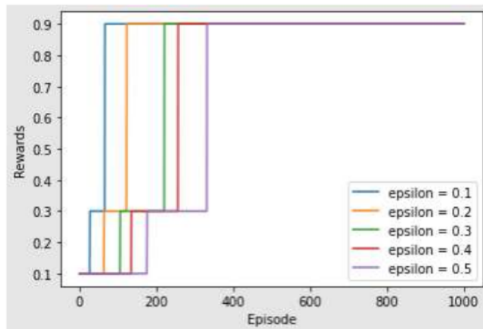
Gambar 6. Hasil Simulasi Kondisi Low Noise
