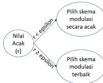
Gambar 3. Cara Kerja Algoritma Epsilon Greedy
