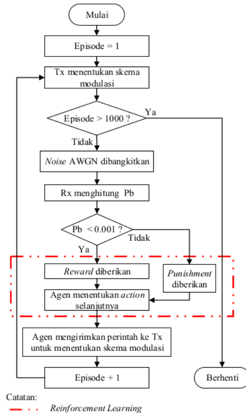
Gambar 4. Alur Simulasi
