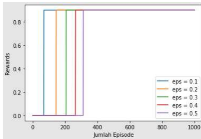
Gambar 8. Hasil Simulasi Kondisi High Noise
