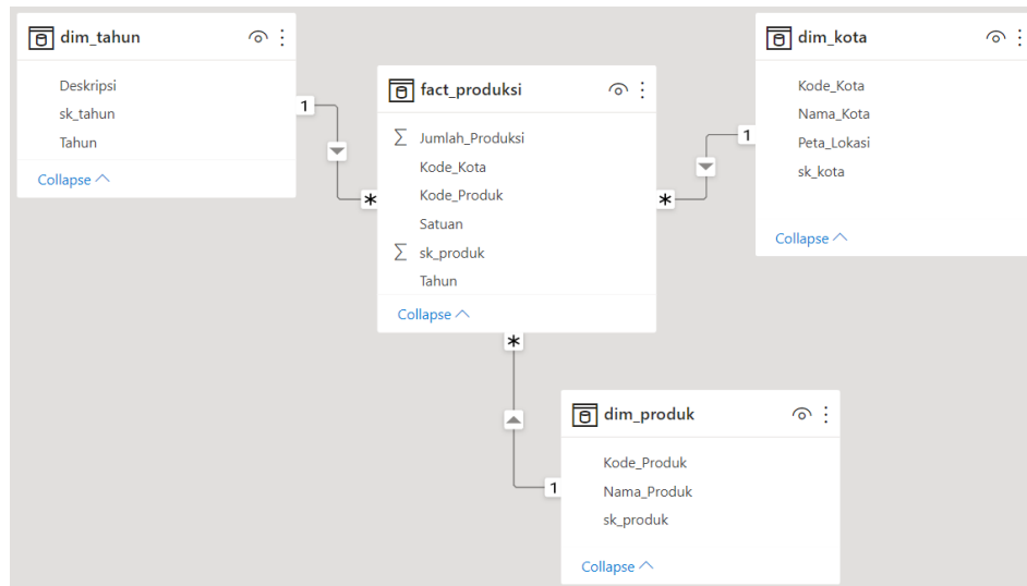
Gambar 5. Diagram Bintang fact_ produksi
