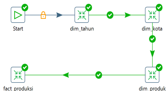
Gambar 9. Job Produksi Tanaman Obat
