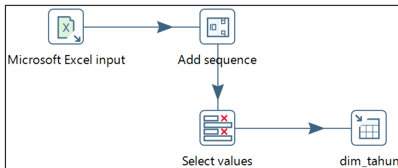
Gambar 6. Transformasi dim_tahun
