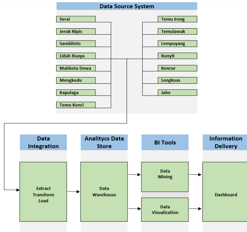
Gambar 2. Arsitektur Sistem Intelijensia Bisnis
