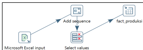
Gambar 8. Transformasi fact_produksi
