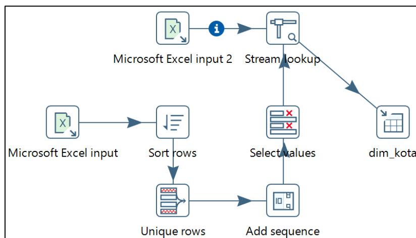
Gambar 7. Transformasi dim_kota
