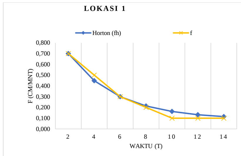
Gambar 5. Grafik laju infiltrasi di lapangan berdasarkan Model Horton
