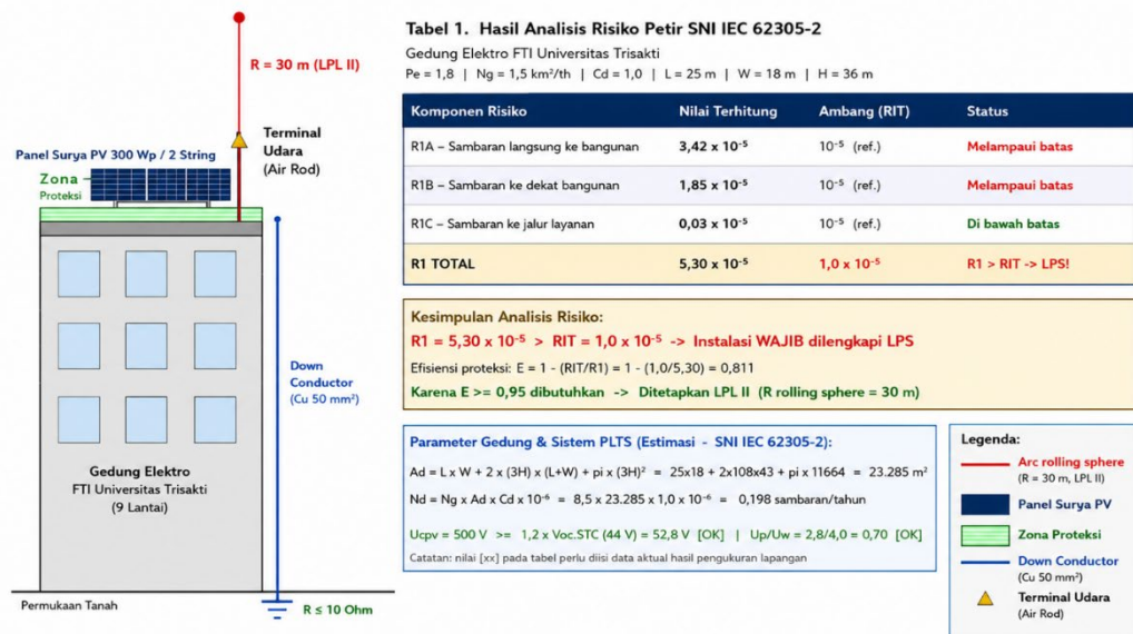
Gambar 1: Ilustrasi penerapan metode rolling sphere pada simulasi zona proteksi terminal udara PLTS rooftop.
