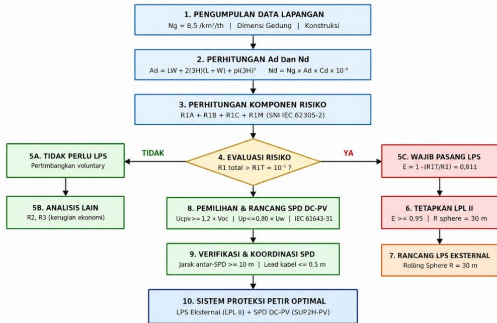
Gambar 2: Alur analisis risiko petir berbasis SNI IEC 62305-2 PLTS rooftop.
