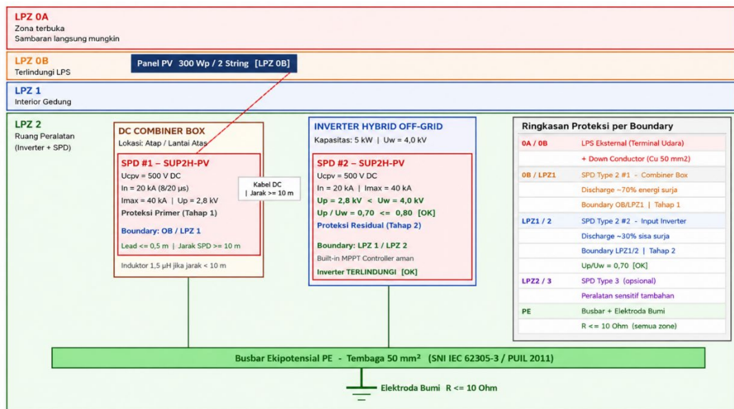
Gambar 3: Konsep zona proteksi petir (Lightning Protection Zone, LPZ) pada sistem PLTS rooftop.
