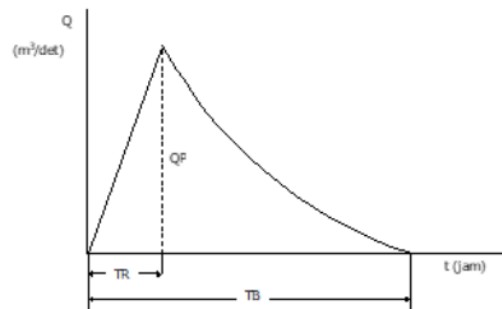
Gambar 2 Sketsa Hidrograf Satuan Sintetik Gama
