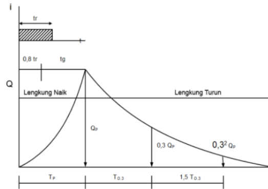
Gambar 1 Sketsa Perhitungan Hidrograf Satuan Sintetik Nakayasu
