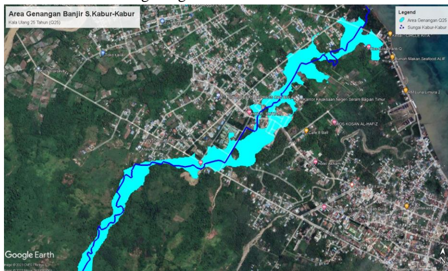
Gambar 7 Hasil Pemodelan Genangan Sungai Kabur-Kabur Q25
