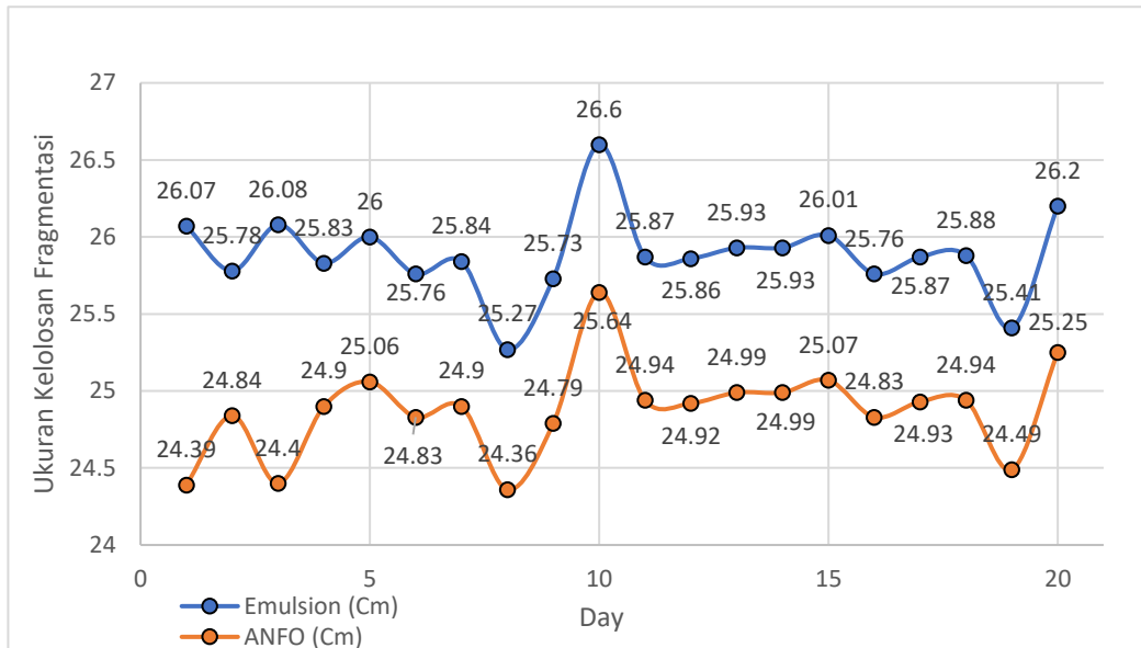
Gambar 2. Grafik Prediksi Fragmentasi Peledakan dengan Kuz-Ram
