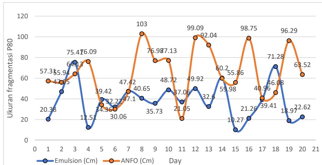
Gambar 3. Fragmentasi Peledakan dengan Menggunakan Software Whipfrag
