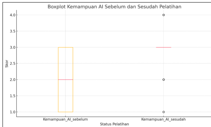
Gambar 3. Visualisasi Boxplot
