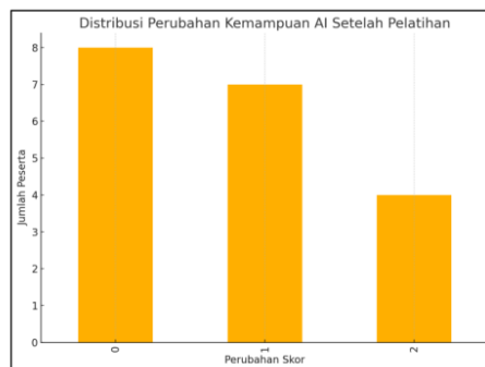
Gambar 2. Visualisasi Deskriptif
