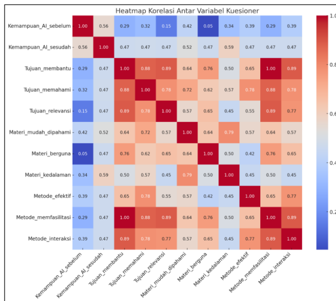
Gambar 4. Visualisasi Heatmap
