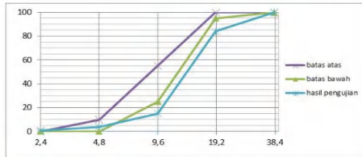
Gambar 4. Gradasi agregat kasar.
