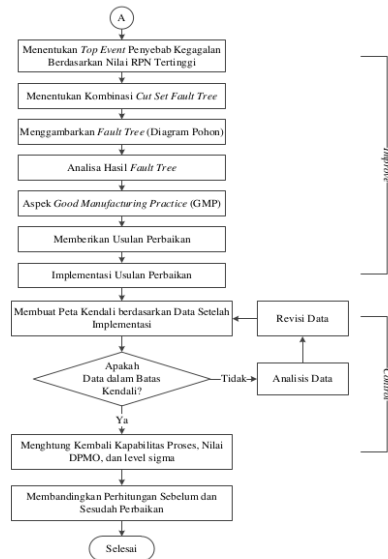
Gambar 3. Flowchart pengolahan data FTA
