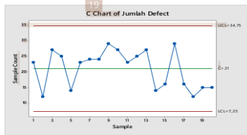
Gambar 4. Peta kendali C bulan Juni 2022
