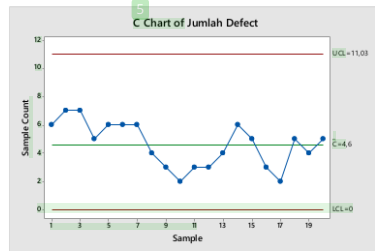
Gambar 17. Peta Kendali C setelah implementasi
