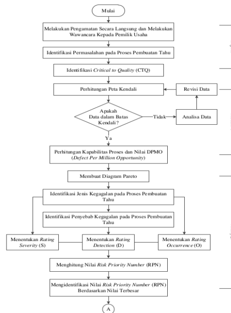
Gambar 2. Flowchart Pengolahan Data FMEA
