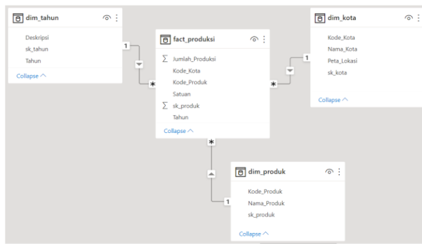
Gambar 5. Diagram Bintang fact_produksi
