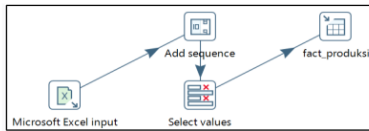
Gambar 8. Transformasi fact_produksi
