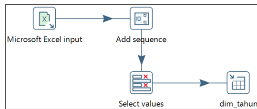
Gambar 6. Transformasi dim_tahun
