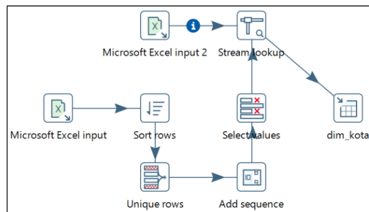
Gambar 7. Transformasi dim_kota
