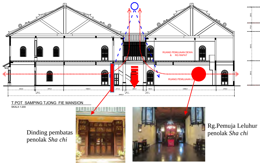
Gambar 4.37 Analisis Fungsi Courtyard terhadap aliran Shen Chi dan Sha Chi Sumber: Penulis 2019
