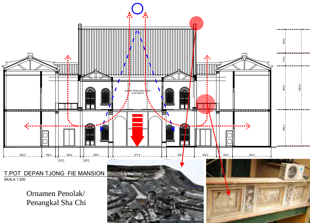
Gambar 4.38 Analisis Fungsi Courtyard terhadap aliran Shen Chi dan Sha Chi Sumber : Penulis 2019
