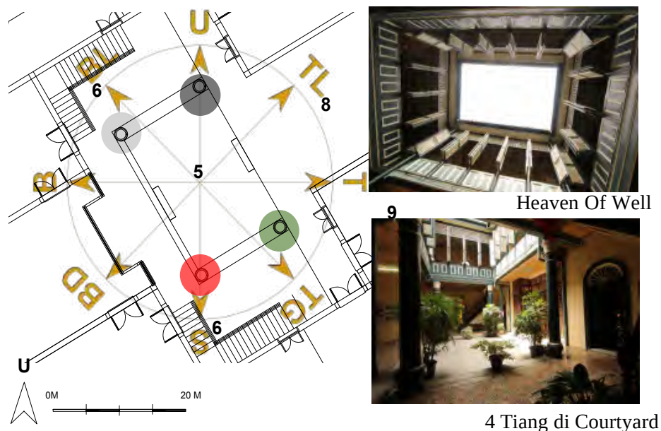
Gambar 4.32 Analisis Tiang Courtyard sebagai Orientasi Ruang /Arah Sumber: Penulis 2019
