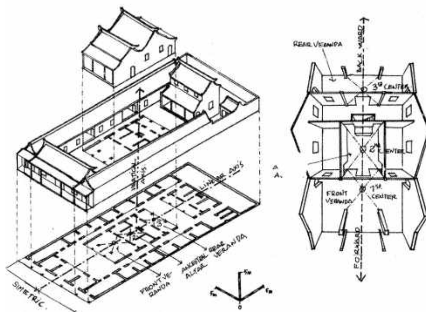
Aksis dan tiga pusat
