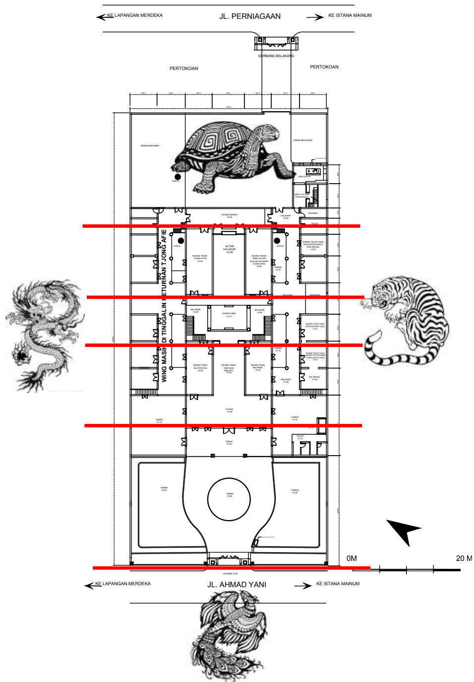
Gambar 4.40 Dinding Pembatas Melintang di kuadran harimau putih dan naga hijau
