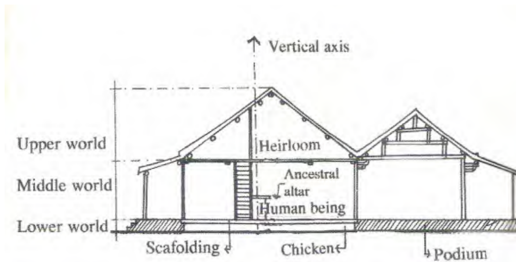
Aksis vertikal dan tiga tingkat kosmos rumah
