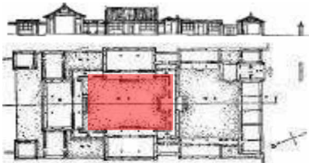
Gambar 2.27 Siteplan Rumah di Peking Sumber: Boyd, 1962, dalam Yi dan Bozovic, 2004
