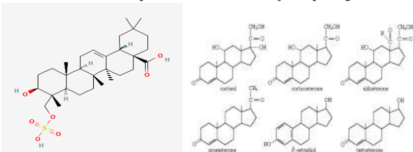
Gambar 34. Struktur triterpenoid dan steroid. A. Triterpenoid. B. Steroid. Sumber: PubChem (2024).
