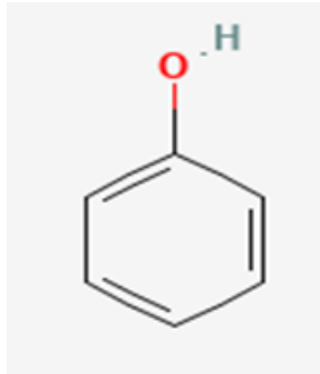
Gambar 38. Struktur fenol. Sumber: Pubchem (2024)
