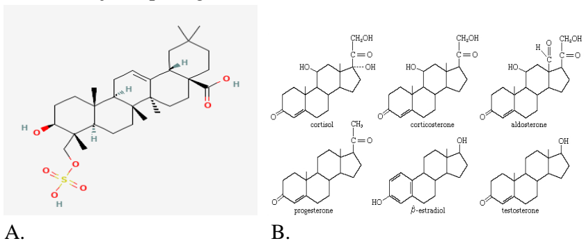
Gambar 34. Struktur triterpenoid dan steroid. A. Triterpenoid. B. Steroid. Sumber: PubChem (2024).
