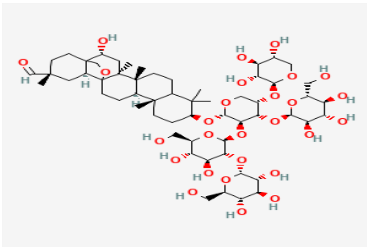
Gambar 37. Struktur saponin. Sumber: Pubchem (2024).
