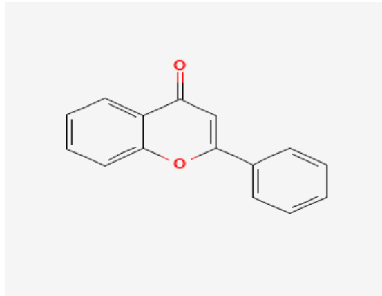
Gambar 36. Struktur flavonoid. Sumber: Pubchem (2024).
