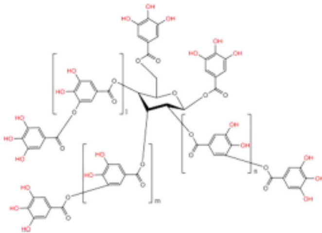
Gambar 35. Rumus struktur steroid. Sumber: Kiechel & Schauer, 2013.
