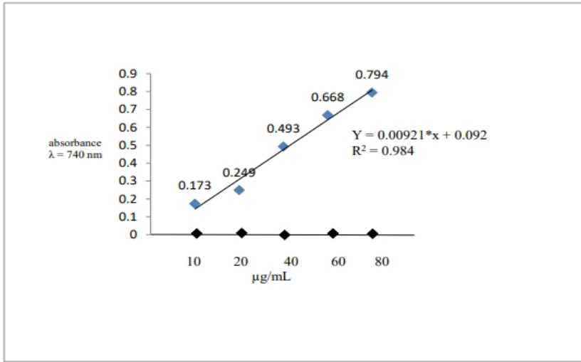
Gambar 47. Kurva standar untuk mengukur kadar tanin ekuivalen asam tanat (TEAT) dalam ekstrak daun L. camara Linn.
