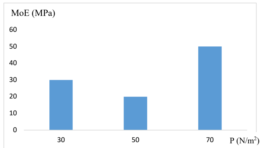
Gambar 3. Modulus elastisitas briket
