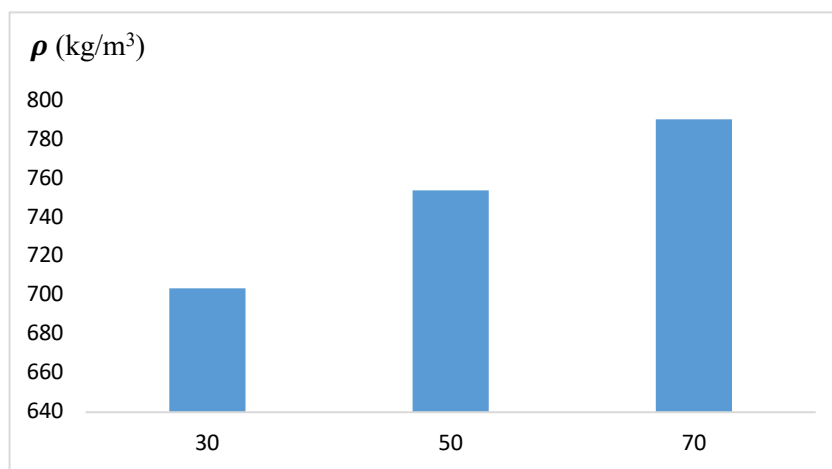
Gambar 1. Pengaruh Tekanan Pembriketan terhadap Densitas Briket
