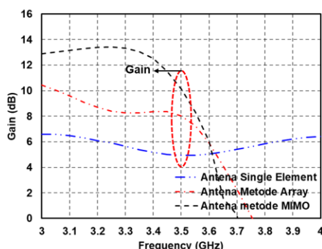
Gambar-16. Perbandingan hasil simulasi gain antenna.
