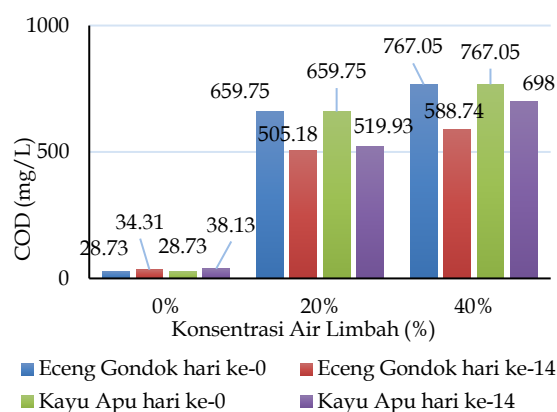
Gambar 6. Pengaruh limbah batik dengan tanaman eceng gondok dan kayu apu terhadap konsentrasi COD (Sumber: Penelitian, 2016)
