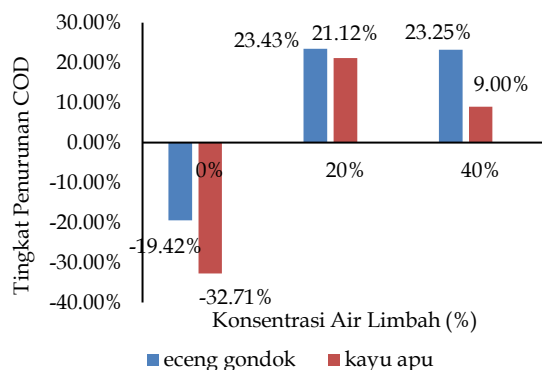
Gambar 7. Penurunan konsentrasi COD pada konsentrasi air limbah dengan eceng gondok dan kayu apu (Sumber: Penelitian, 2016)
