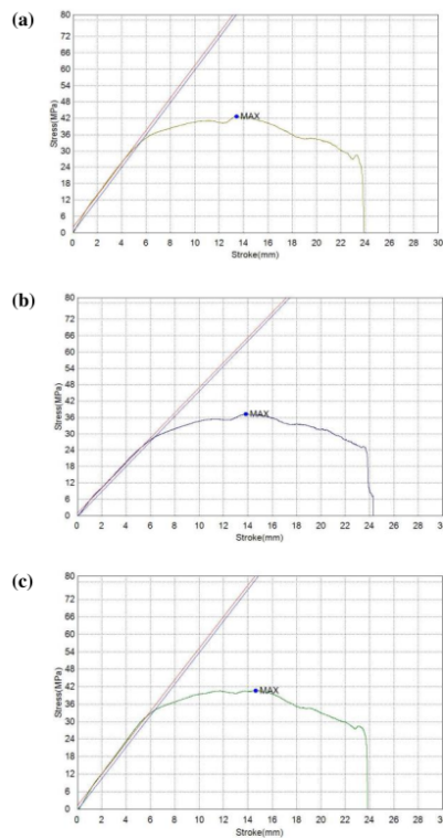
Gambar 2. Grafik hasil uji kekuatan fleksural bahan termoplastik nilon (a) perendaman dengan akuades, (b) perendaman dengan obat kumur I, (c) perendaman dengan obat kumur II
