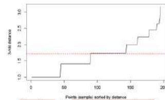
Gambar 5. K-dist dengan k = 5
