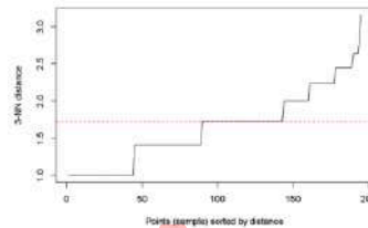
Gambar 3. K-dist dengan k = 3
