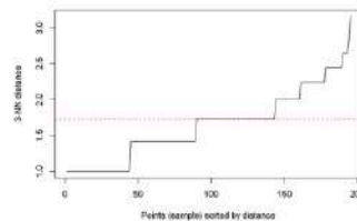
Gambar 4. K-dist dengan k = 4
