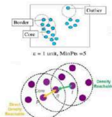
Gambar 1. Terminologi dalam Algoritma DBSCAN
