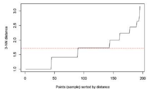
Gambar 4. K-dist dengan k = 4
