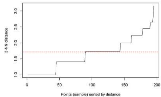
Gambar 3. K-dist dengan k = 3
