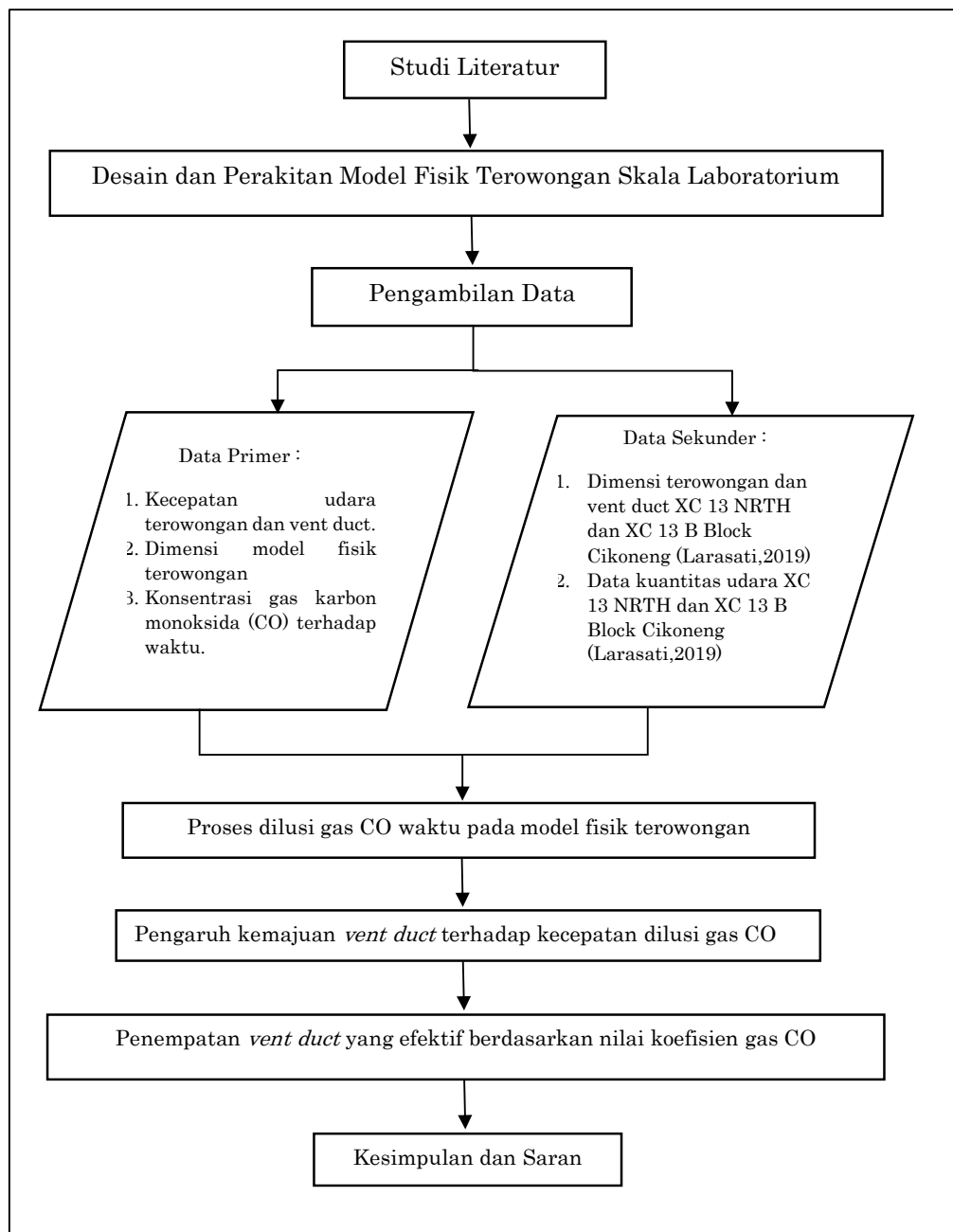
Gambar 1. Tahapan Penelitian
