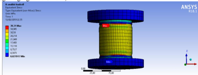
Gambar 2. Simulasi tegangan maksimal yang diterima load cell
