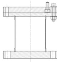
Gambar 1. Rancangan bentuk dinamometer
