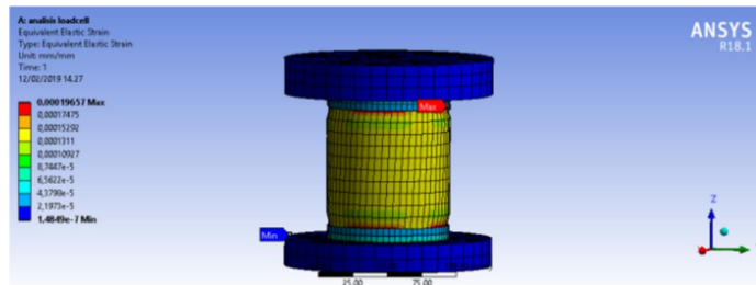
Gambar 3. Simulasi regangan maksimal yang diterima load cell
