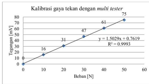
Gambar 9. Kalibrasi gaya tekan dengan multi tester
