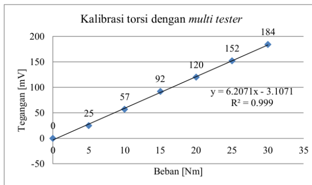
Gambar 10. Kalibrasi momen puntir dengan multi tester
