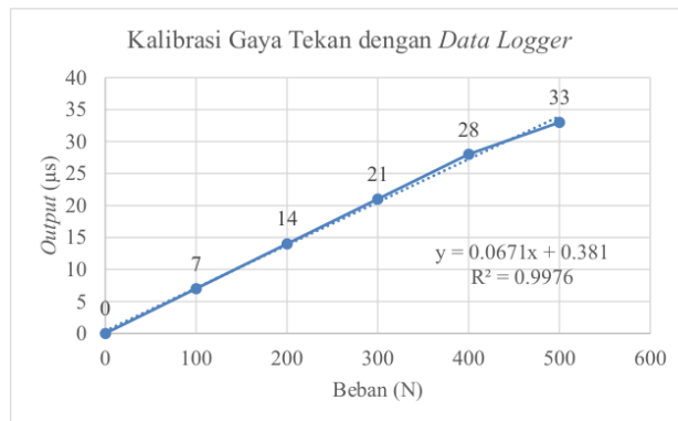
Gambar 7. Grafik kalibrasi gaya tekan
