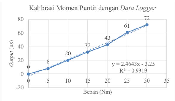
Gambar 8. Grafik kalibrasi momen puntir
